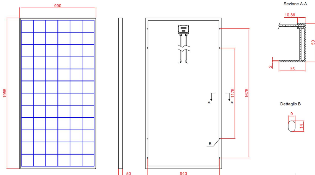
DISEGNO TECNICO / TECHNICAL DRAWING
